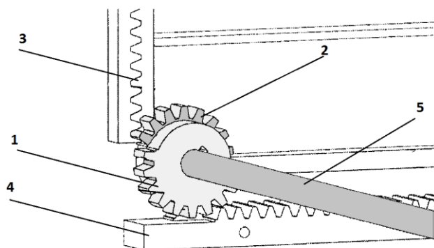
Rys. 1. Mechanizm koła zębatego.
